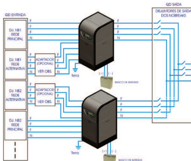
TOP-DSP Paralelo Ativo-CE COM com entrada principal e rede alternativa
