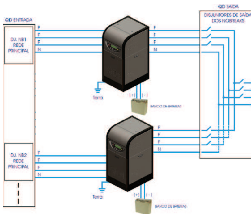
TOP-DSP Paralelo Ativo-CE COM com entrada principal e rede alternativa interna.
